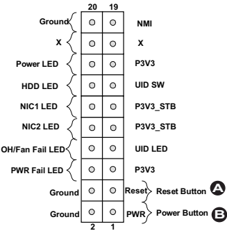
A. Reset Button B. PWR Button
