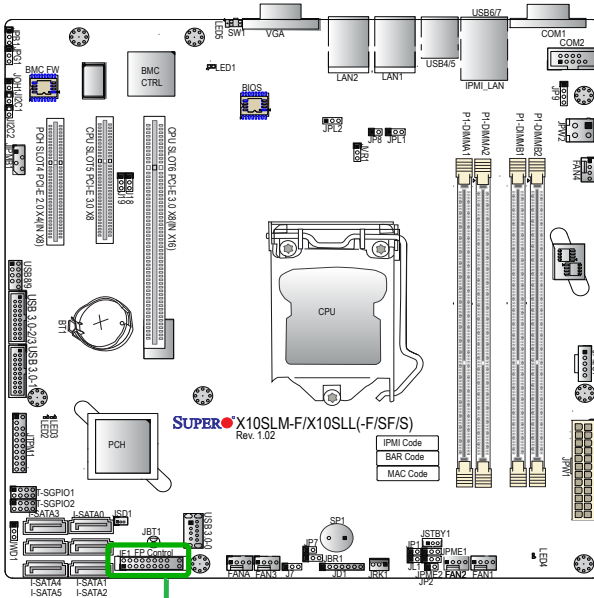
JF1 Header Pins
